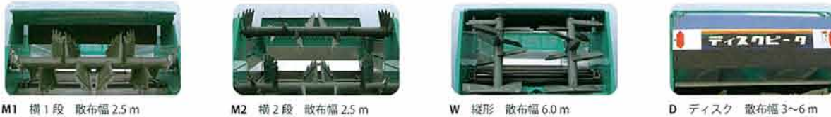
M1 横1段 散布幅 2.5 m M2 横2段 散布幅 2.5 m W 縦形 散布幅 6.0 m D ディスク 散布幅 3~6 m
