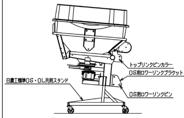
組付け完成図 (日農工標準オートヒッチO・I)
