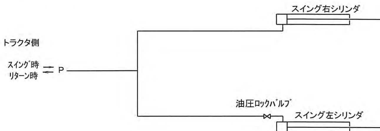
スイングシリンダ油圧回路図
