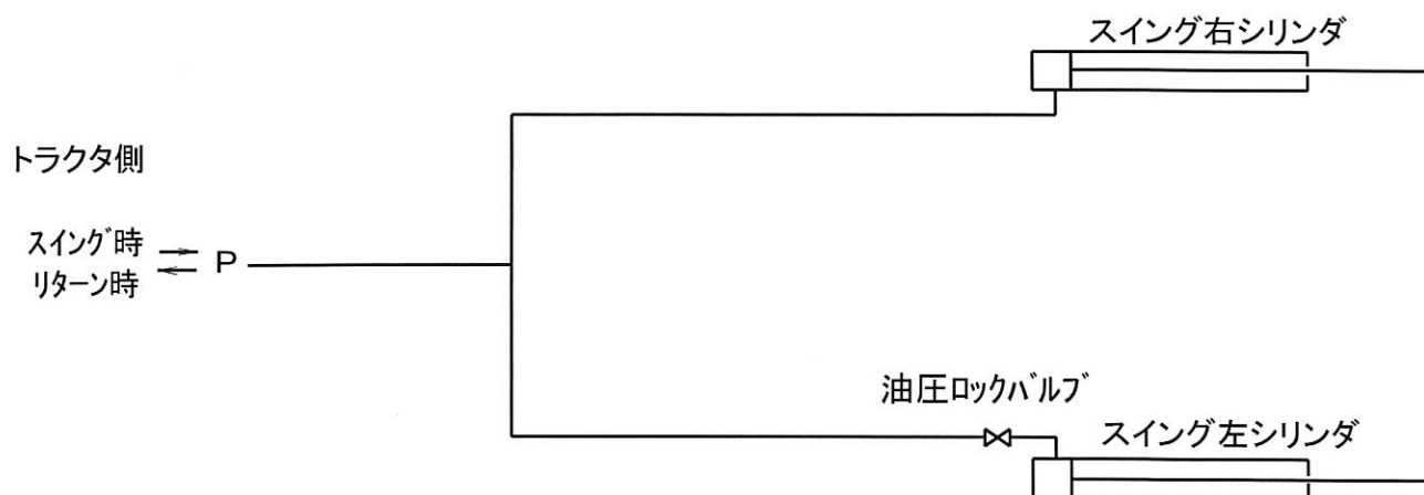
スイングシリンダ油圧回路図
