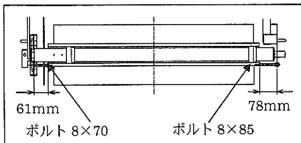
正面視
