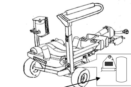
車台番号打刻位置 シャーシ右後方
